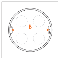
B. \Phi 60 mm priemer inštaláčnej krabičky KPR 68 od skrutky po skrutku.
